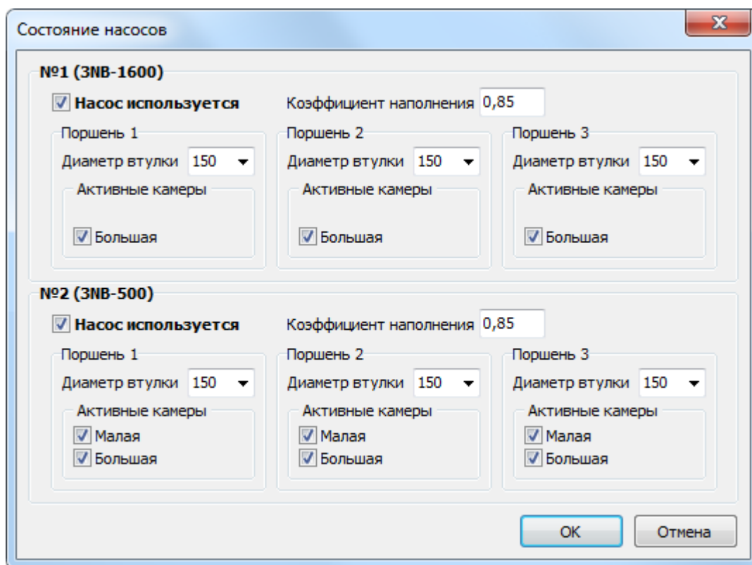
Рисунок 77. Состояние насосов
