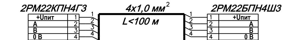
Рисунок А.3 – Схемы подключения РУД-342 к компьютеру (при использовании УРСК):
